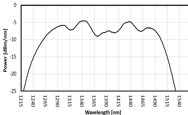
FIG. 1: OSE2 SPECTRUM
