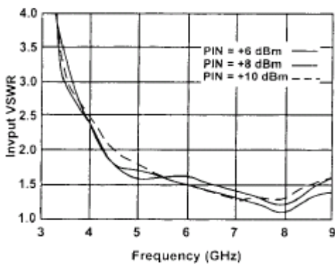
Input VSWR
