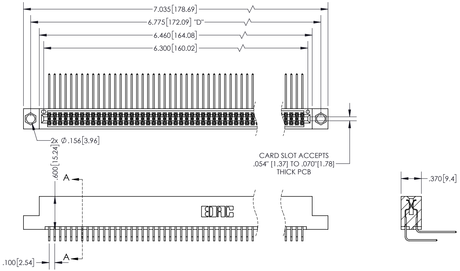
SECTION A-A
