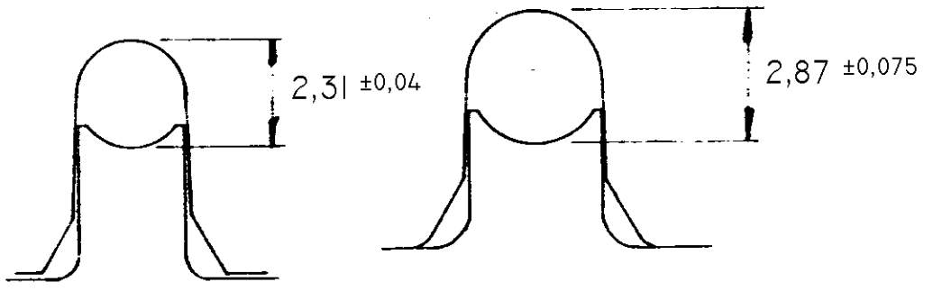
Sertissage isolant
