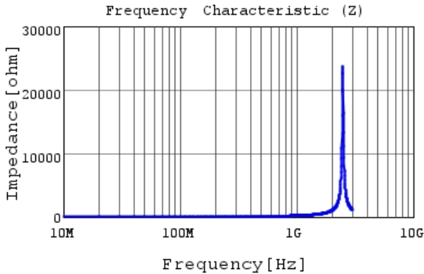
LQG15WH30NH02 |Z|
