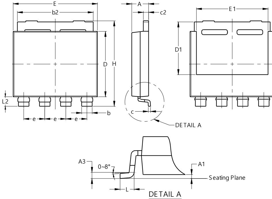
PowerDI8080-5
