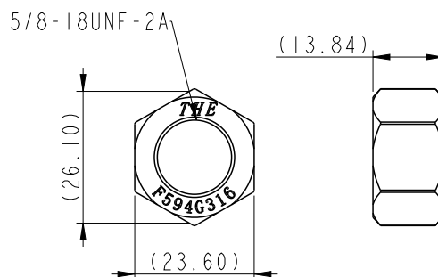
Nut
