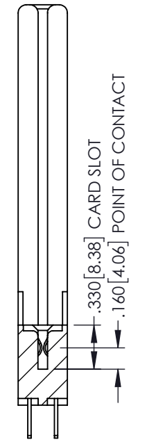
SECTION A-A
