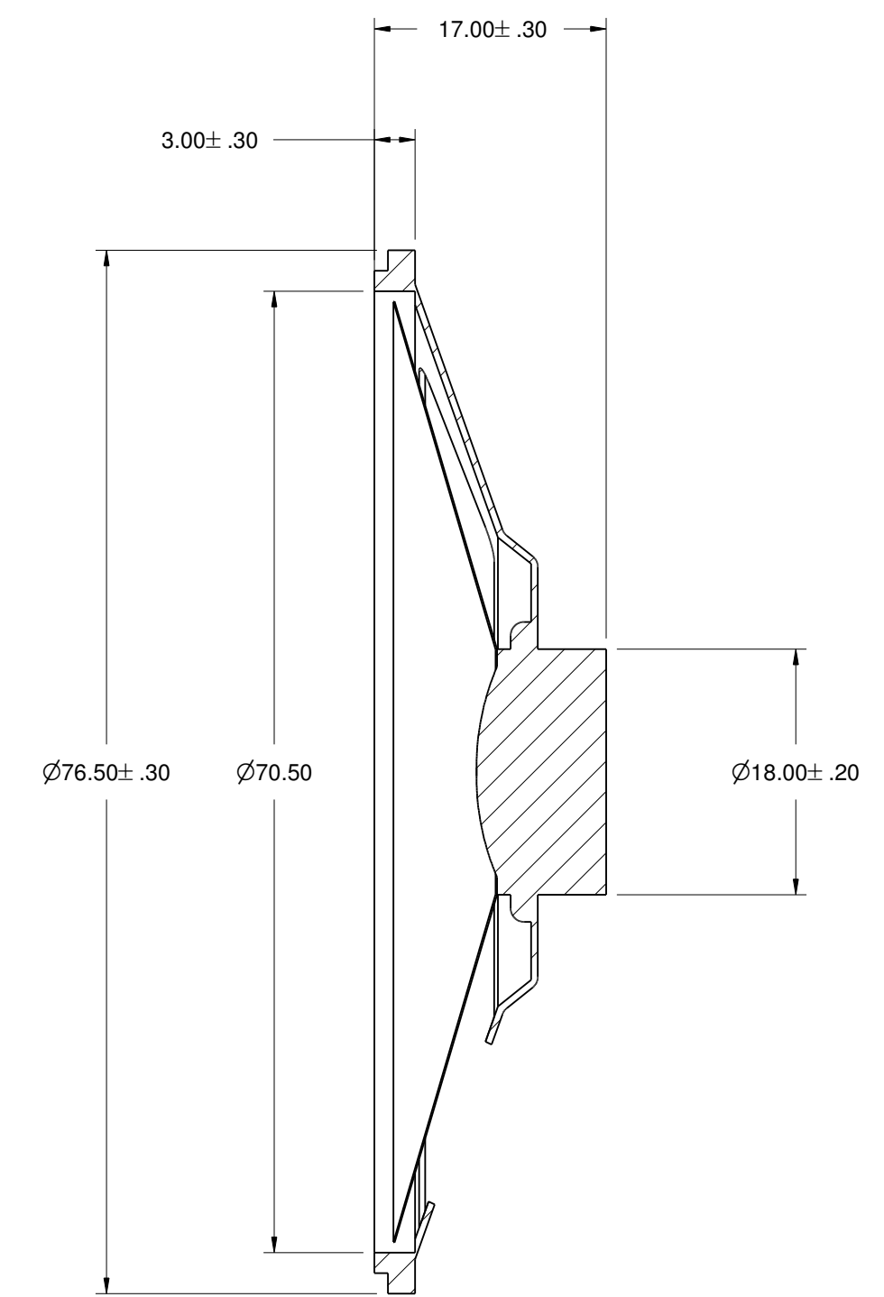
Section A-A
