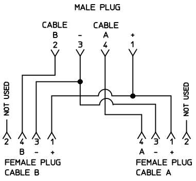
WIRING SCHEMATIC
