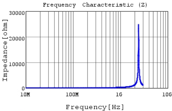
LQG15WZ33NG02 |Z|
