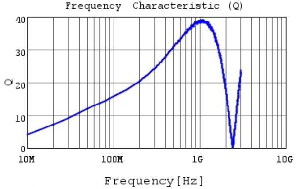
LQG15WZ33NG02 Q
