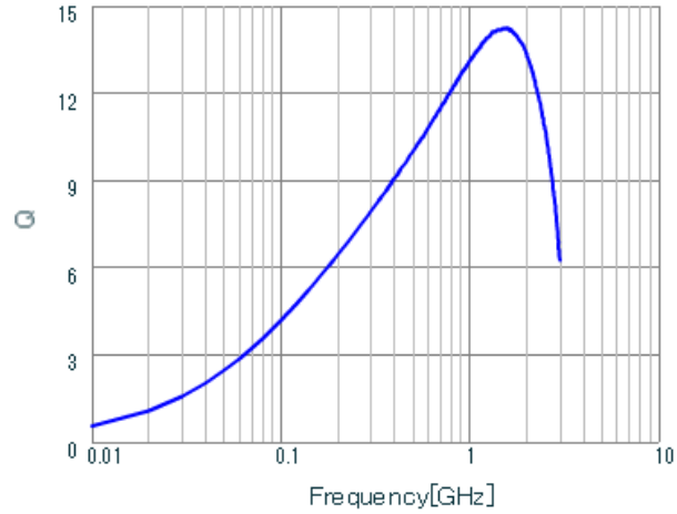
LQP02TN18NH02 Q.
