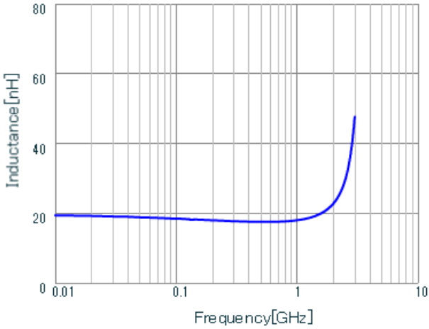
LQP02TN18NH02 L.
