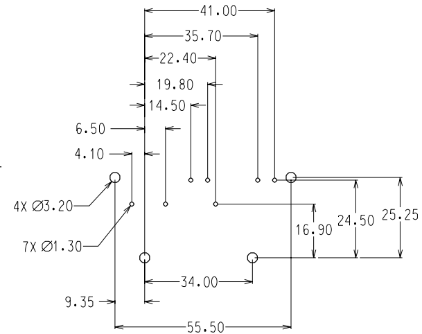
P.C.B. HOLE LAYOUT
