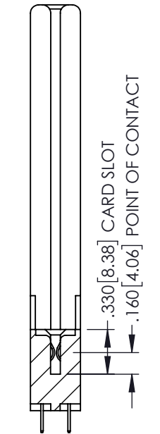
SECTION A-A
