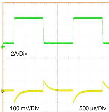
12\text{ V}_{IN} 3.3\text{ V}_O 0.5- to 5-A Step
