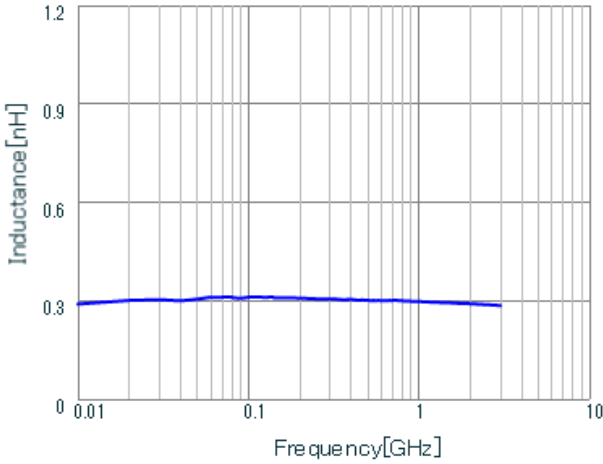
LQP02TQ0N3C02 L.
