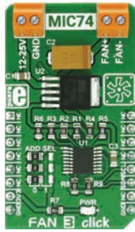
Fan 3 Click
