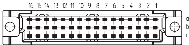
Bestückungsplan / contact layout bestückt / assemble
