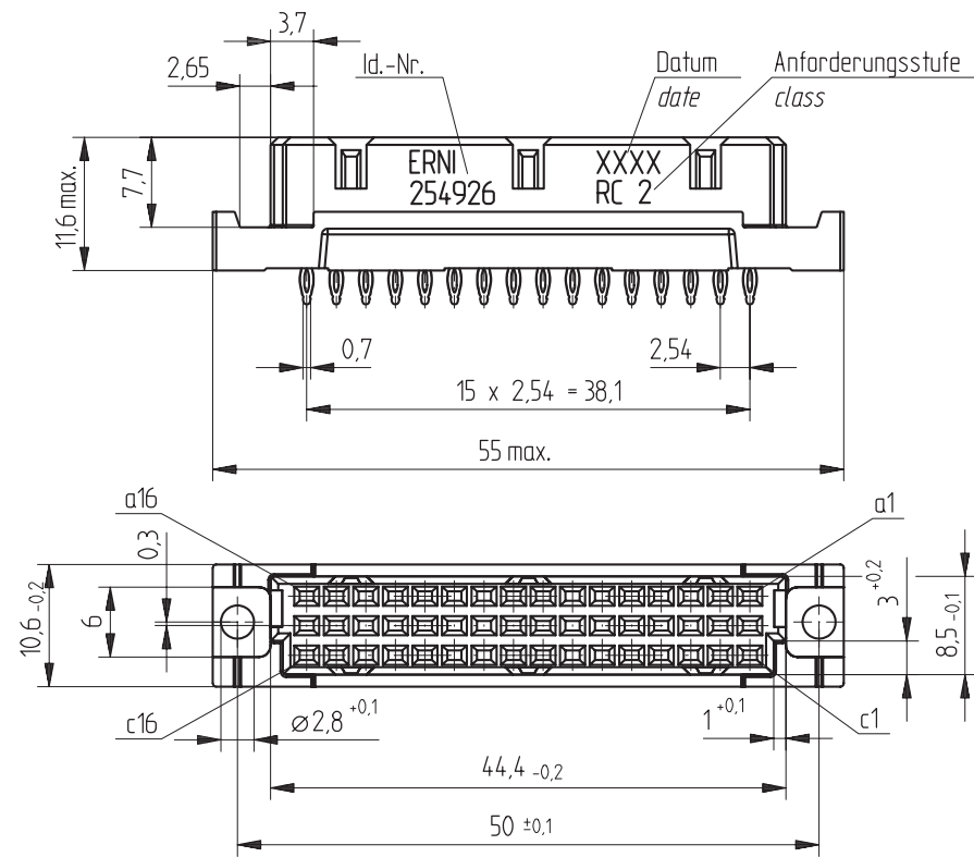
Bestückungsplan / contact layout bestückt / assemble
