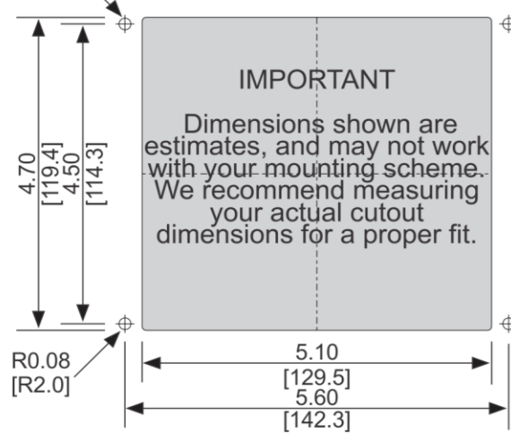
Cutout Dimensions
