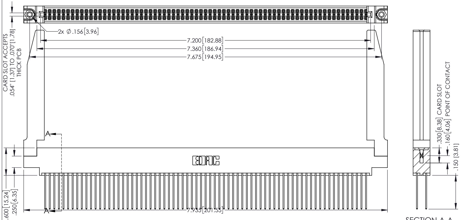
SECTION A-A
