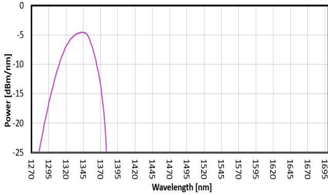
FIG. 7: SLED 6 SPECTRUM
