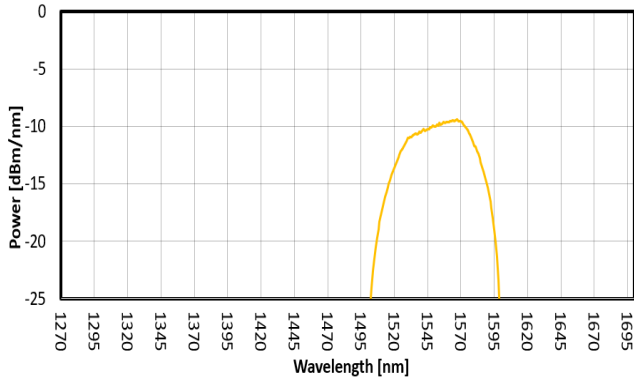
FIG. 3: SLED 2 SPECTRUM
