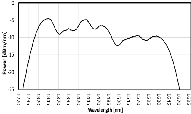
FIG. 1: ISB2 SPECTRUM
