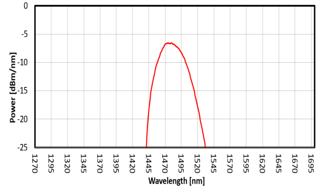
FIG. 4: SLED 3 SPECTRUM
