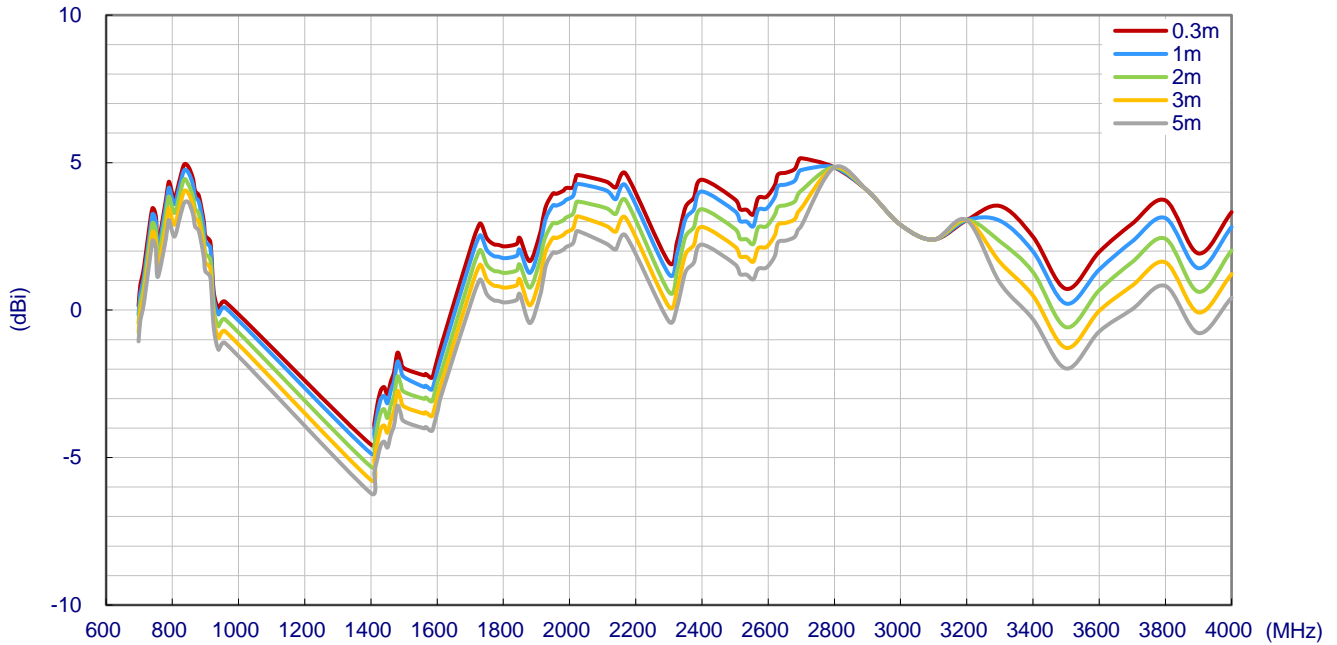
5G/4G MIMO 2
