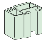
Bar 800 A. LVS04503
