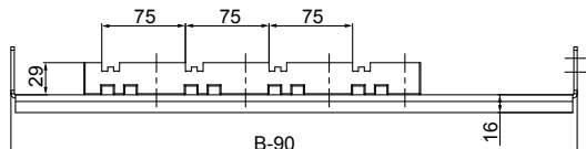
NSYBHS500
