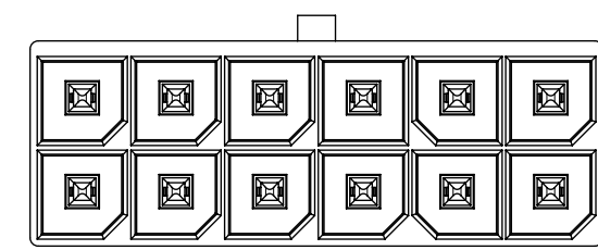
12 CKT
