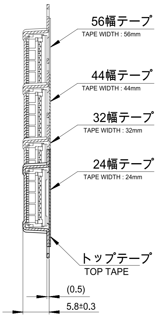
断面 Y-Y SECTION Y-Y
