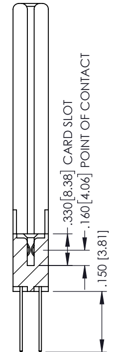
SECTION A-A
