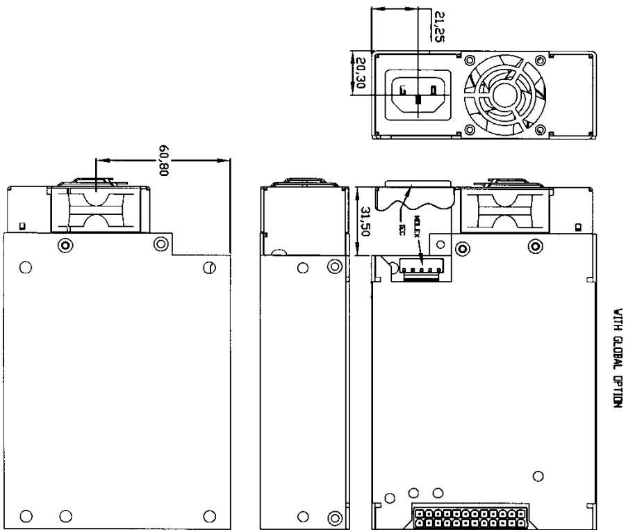
NV175 WITH OPTIONAL CASE & FAN
