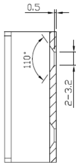
a-a 剖面圖
