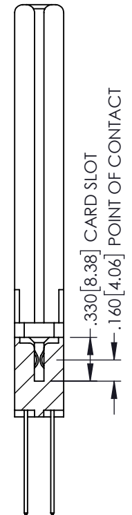
SECTION A-A
