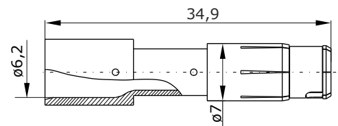
Hauptabmessungen Kontaktbuchse
