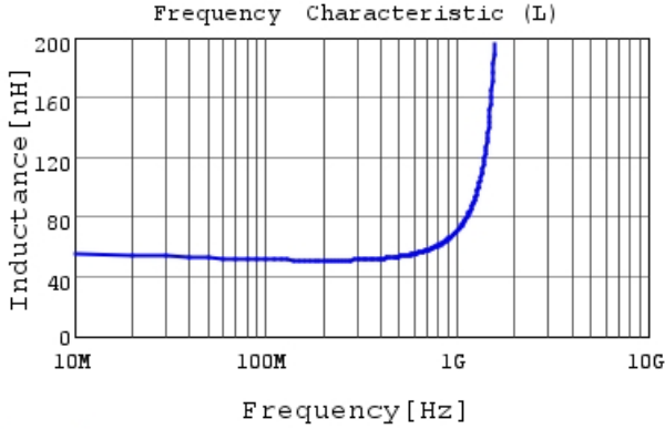
LQG15WH51NH02 L
