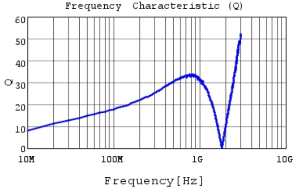
LQG15WH51NH02 Q
