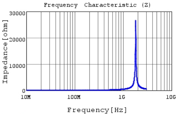
LQG15WH51NH02 |Z|
