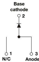
D 2 PAK (TO-263AB)
