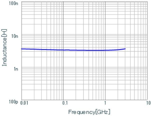
LQG15WZ3N3B02 L.
