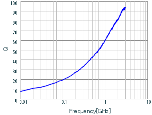
LQG15WZ3N3B02 Q.
