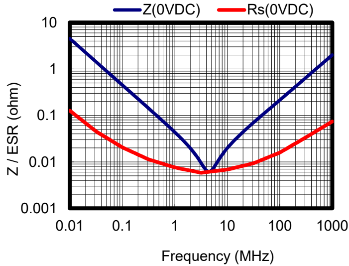
Impedance/ESR
