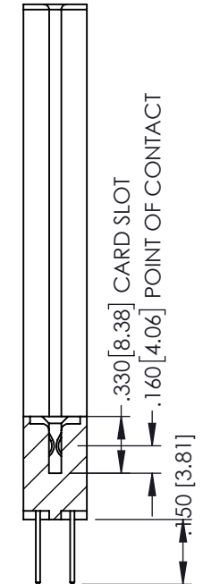
SECTION A-A
