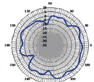
Port 3
