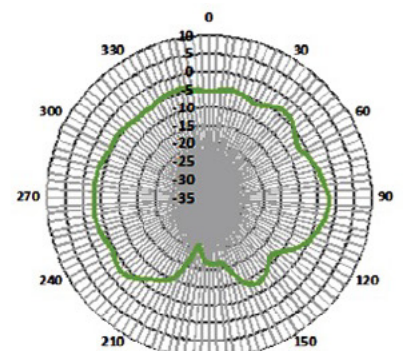
Port 3
