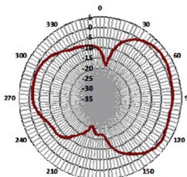
Port 2
