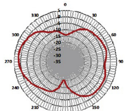
Port 3
