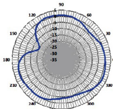
Port 2
