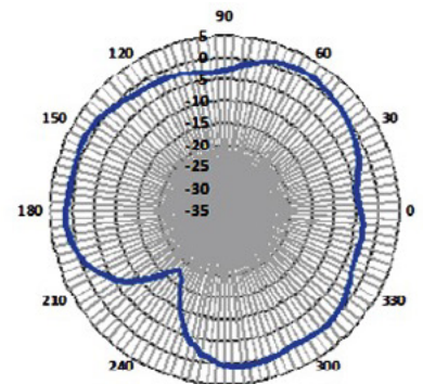
Port 3
