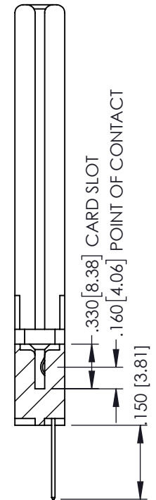
SECTION A-A
