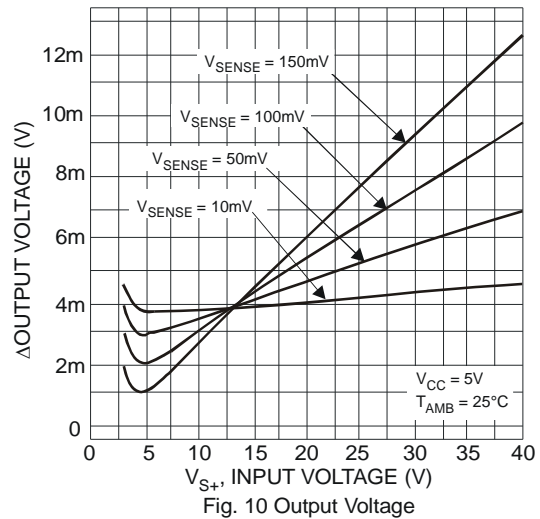
Fig. 10 Output Voltage
