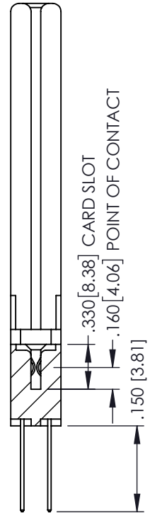
SECTION A-A
