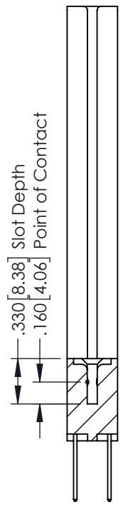
SECTION A-A
