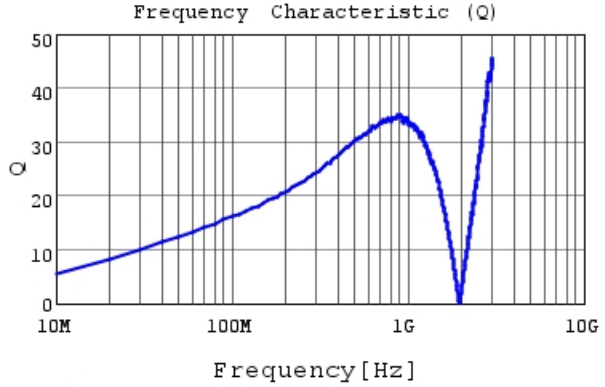
LQG15WH47NG02 Q
