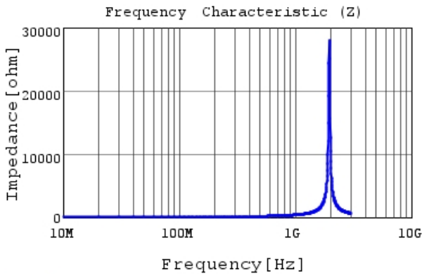
LQG15WH47NG02 |Z|
