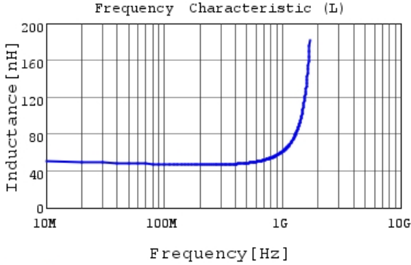
LQG15WH47NG02 L
