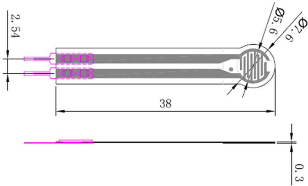
RP-C7.6-LT Dimension Diagram
