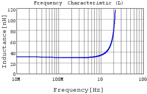
LQG15WZ30NJ02 L
