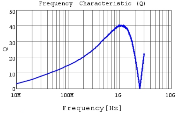
LQG15WZ30NJ02 Q
