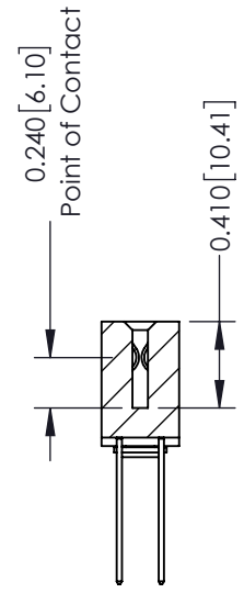
SECTION A-A
