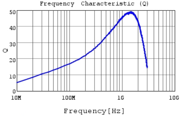
LQG15WZ18NG02 Q
