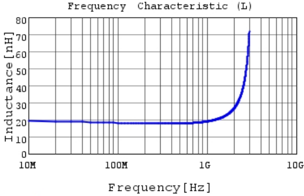
LQG15WZ18NG02 L
