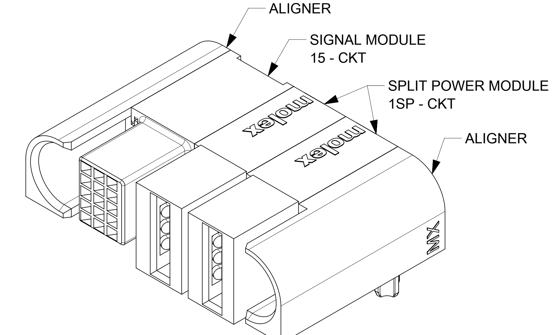
P/N: 171090-8412 (G-2SP-15S-G)
