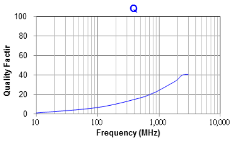
WLCM0603TN□3N6TB
