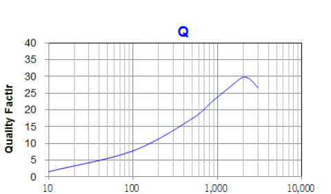
WLCM0603TN□8N2TB
