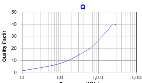
WLCM0603TN□6N8TB
