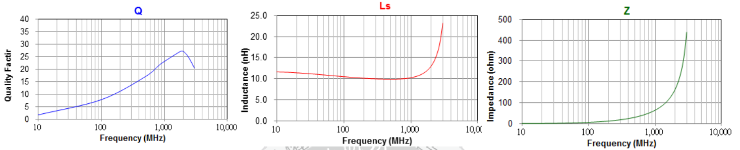
WLCM0603TN□10NTB
