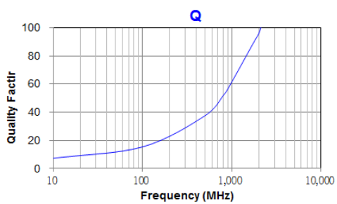
WLCM0603TN□1N0TB
