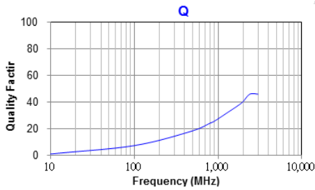
WLCM0603TN□3N8TB
