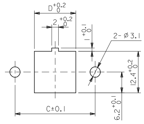
パネル切抜寸法 (参考) PANEL CUT OUT DIM.
