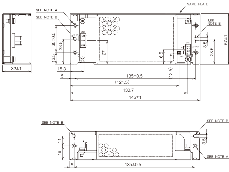
(unit : mm)
