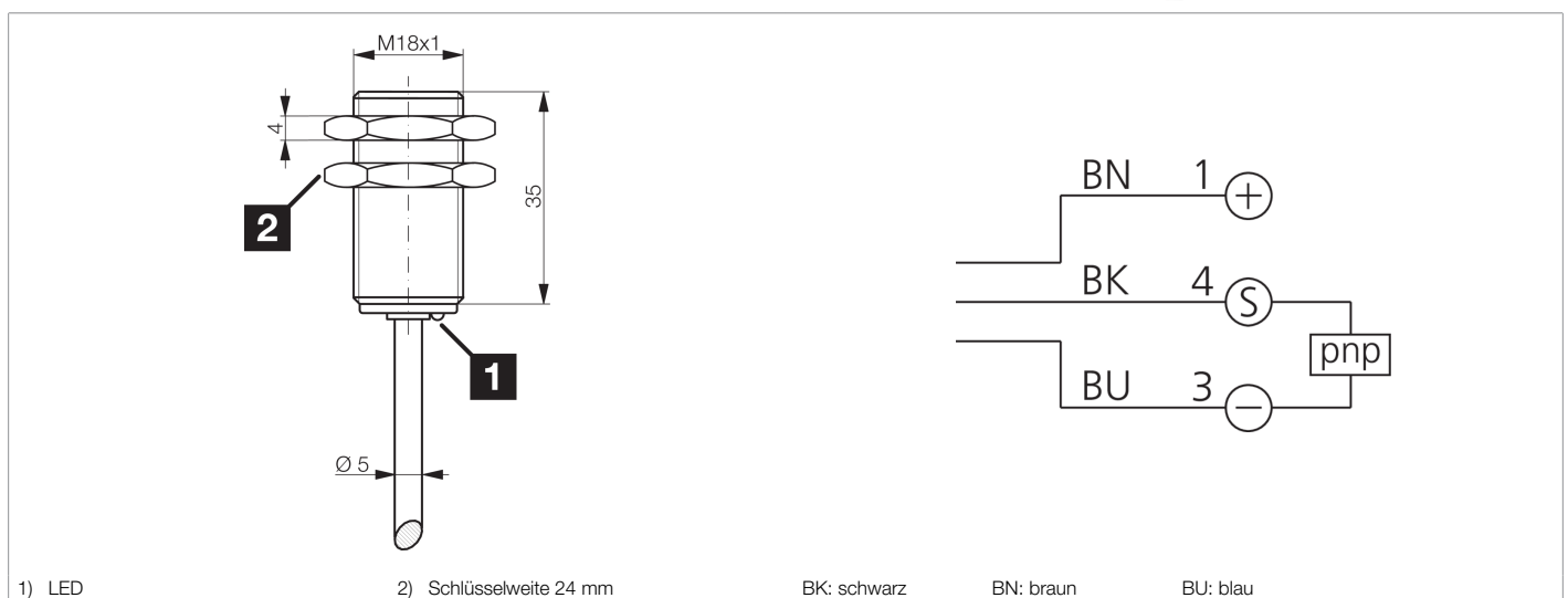
1) LED 2) Schlüsselweite 24 mm BK: schwarz BN: braun BU: blau
